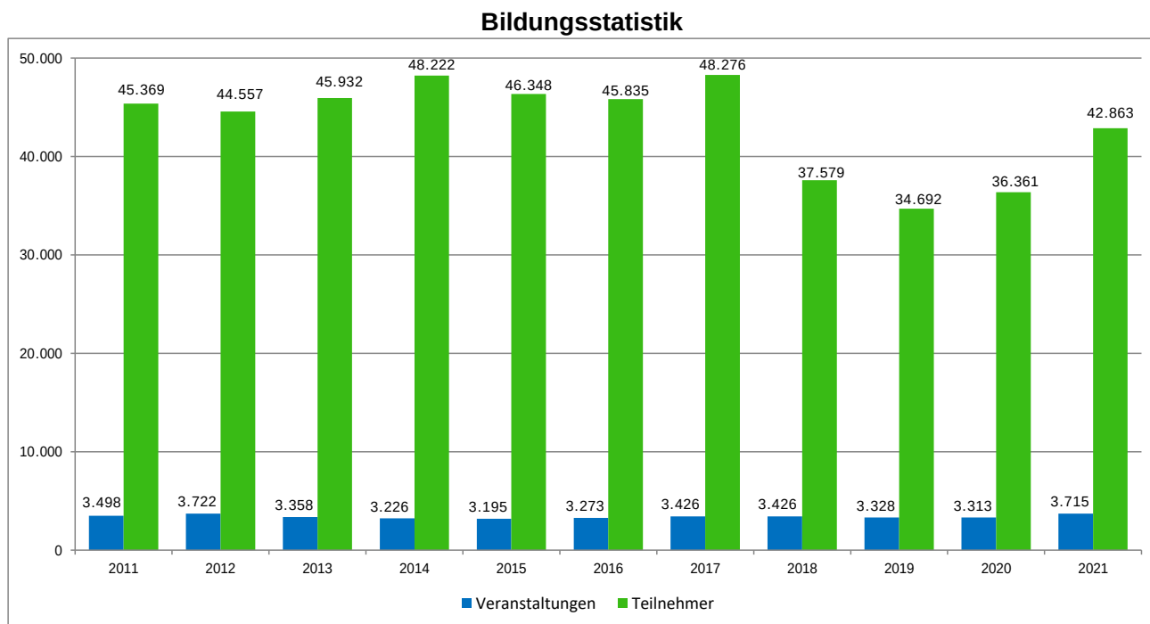
Abb. 7 Bildungsstatistik
