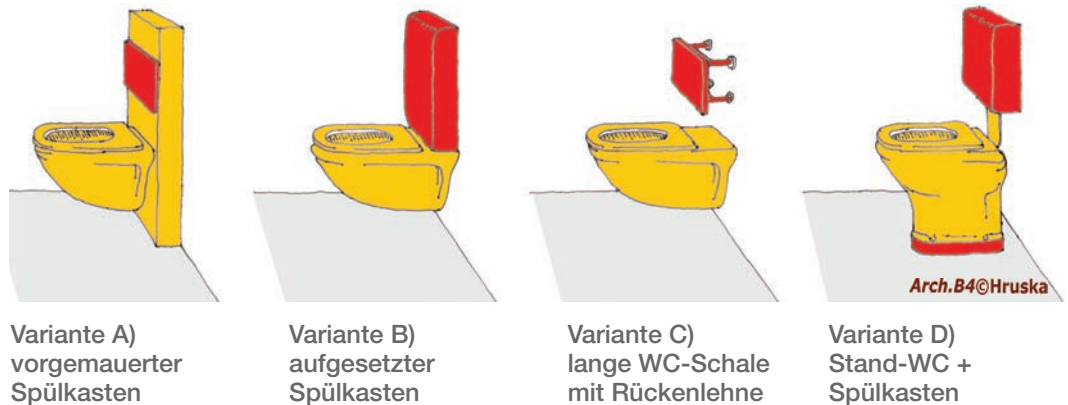
Bild 9: Ausführungsvarianten, WC-Sitz mit Anlehnflächen
