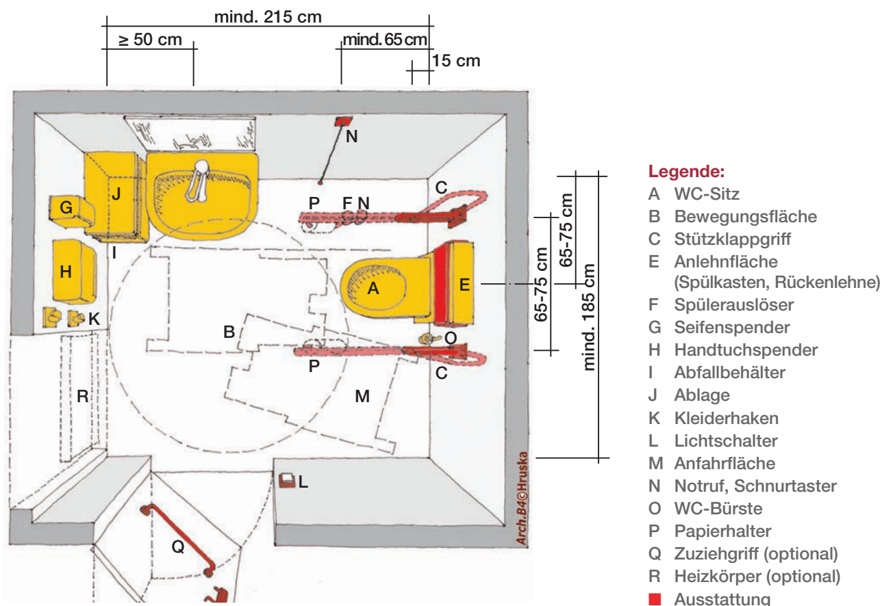
Bild 3: Grundriss zu Bild 1. WC-Anlage mit Handwaschbecken in Mindestgröße
